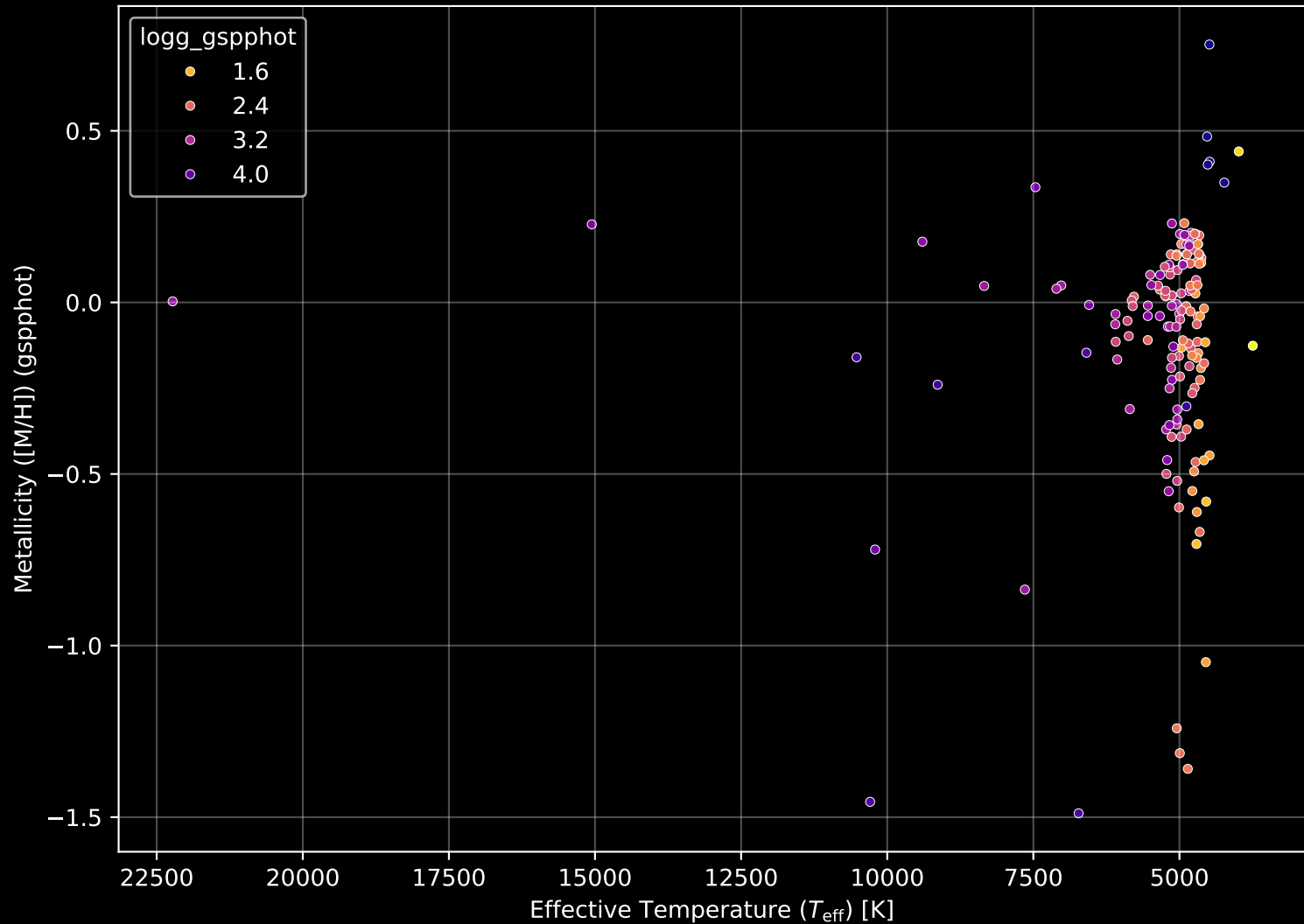
APOGEE DR17 Field: [114-25_btx] Stellar Population Parameters (n= 154)
